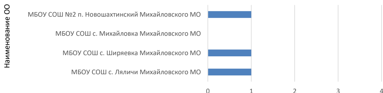
Рис. 1. Количество попаданий ОО в перечни ОО с необъективными результатами по русскому языку в 2022-2025 гг.
