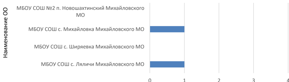
Рис. 2. Количество попаданий ОО в перечни ОО с необъективными результатами по математике в 2022-2025 гг.
